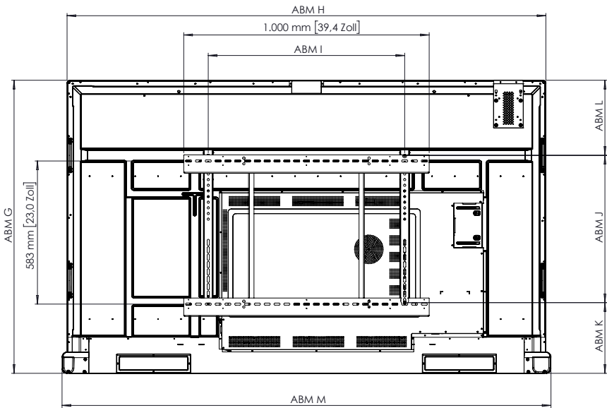
Rückansicht
